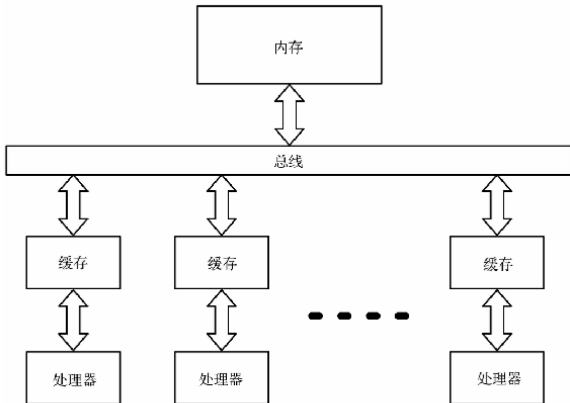
图 1-1 共享内存的多处理器系统
