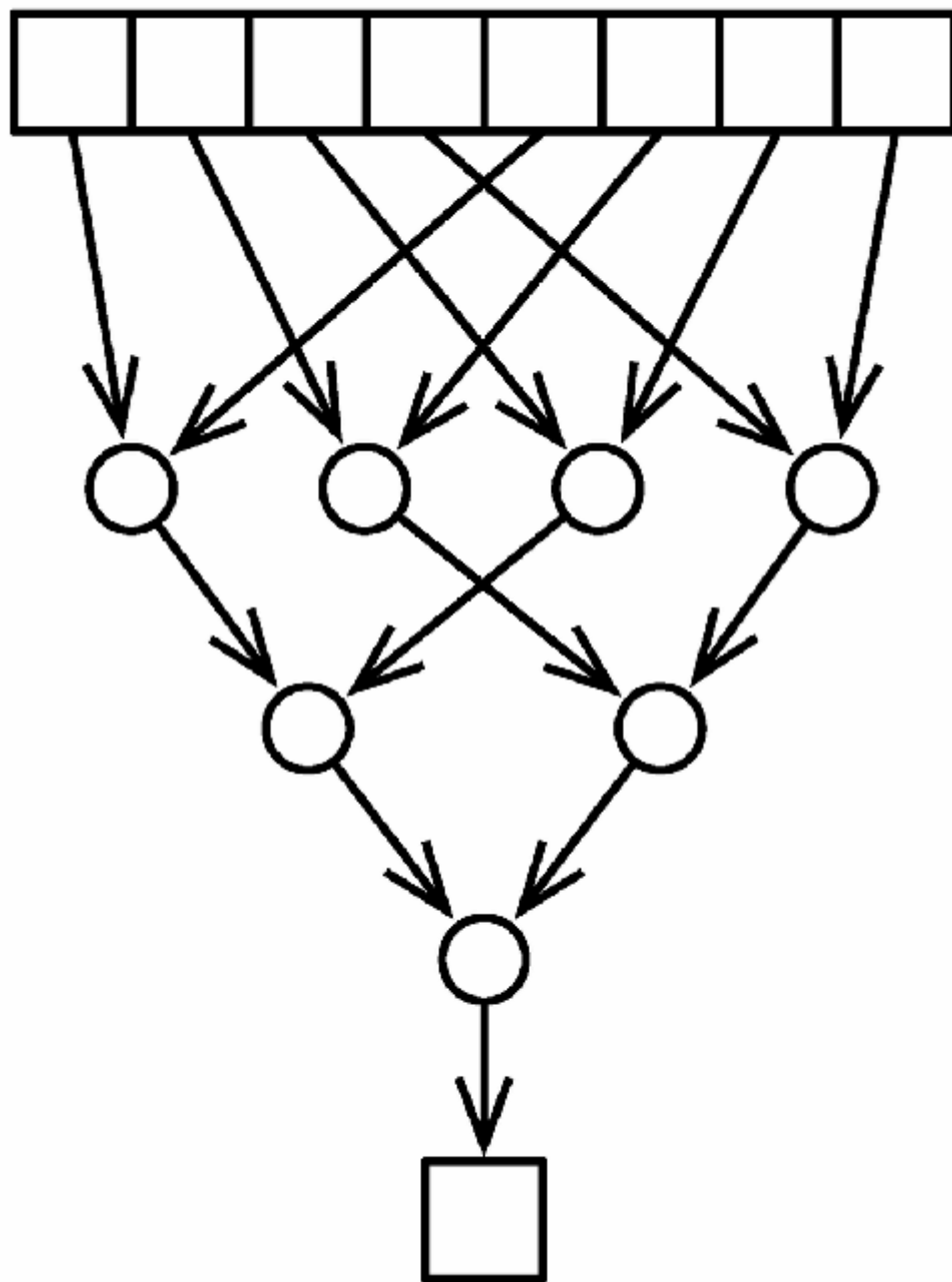
图 7-7 化简操作的树形顺序
