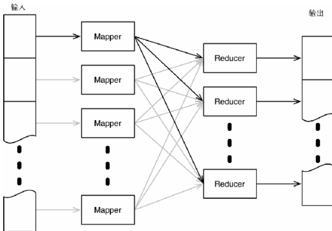
图 8-2 Hadoop数据流
