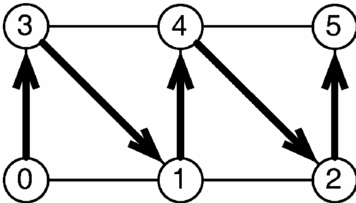
图 7-11 三角形带
