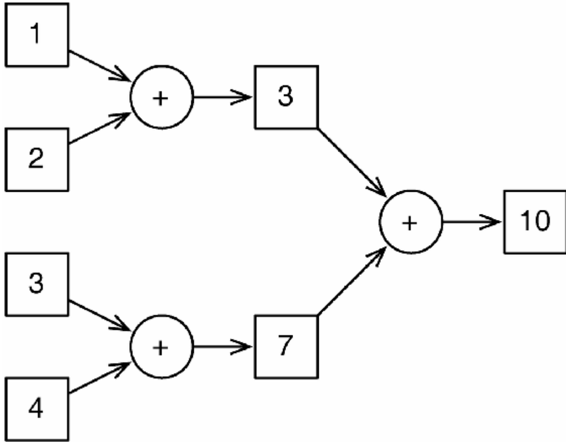
图 3-4 (+ (+ 1 2) (+ 3 4)) 的数据流
