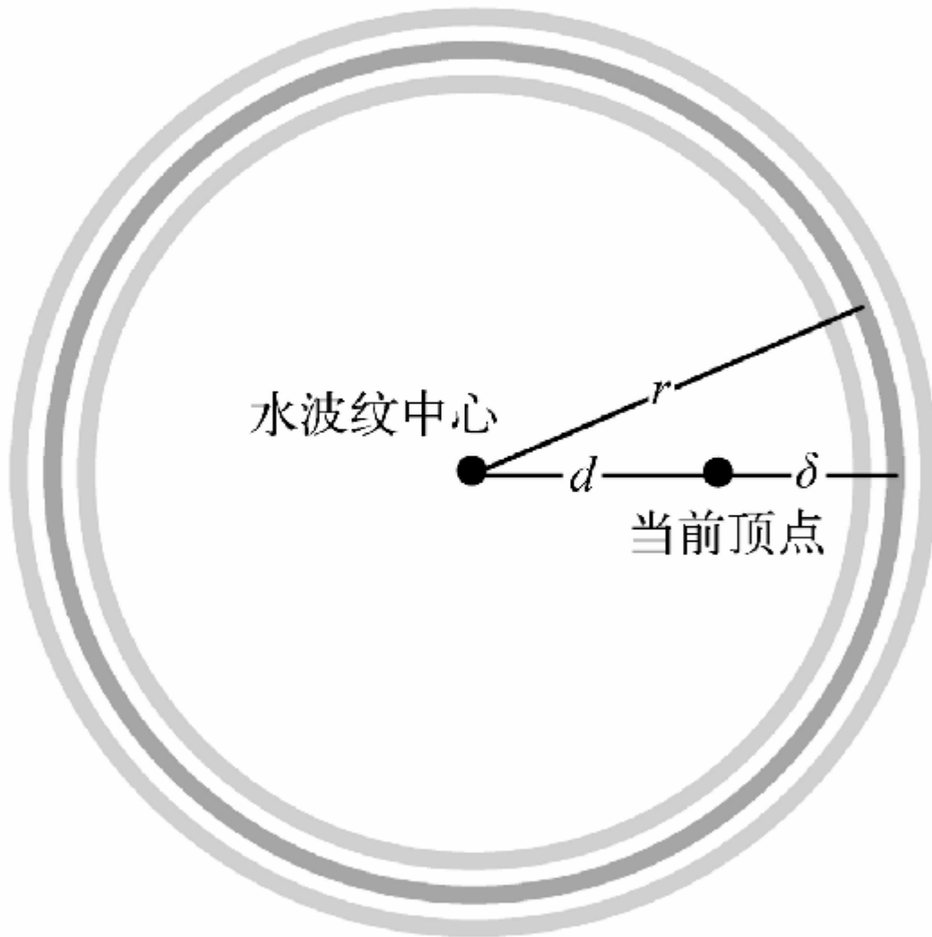
图 7-12 水波纹的参量
