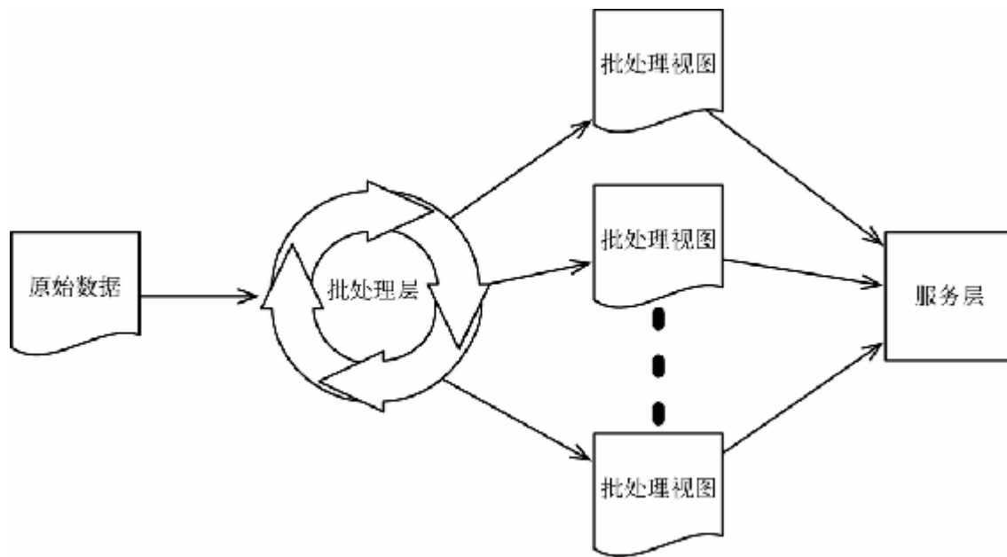
图 8-9 数据系统
