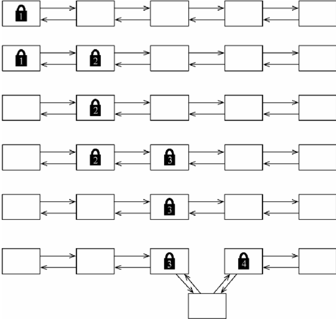
图 2-2 交替锁
