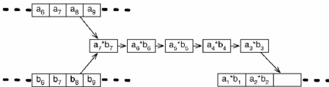
图 7-2 多组数乘法的饱和的操作流水线
