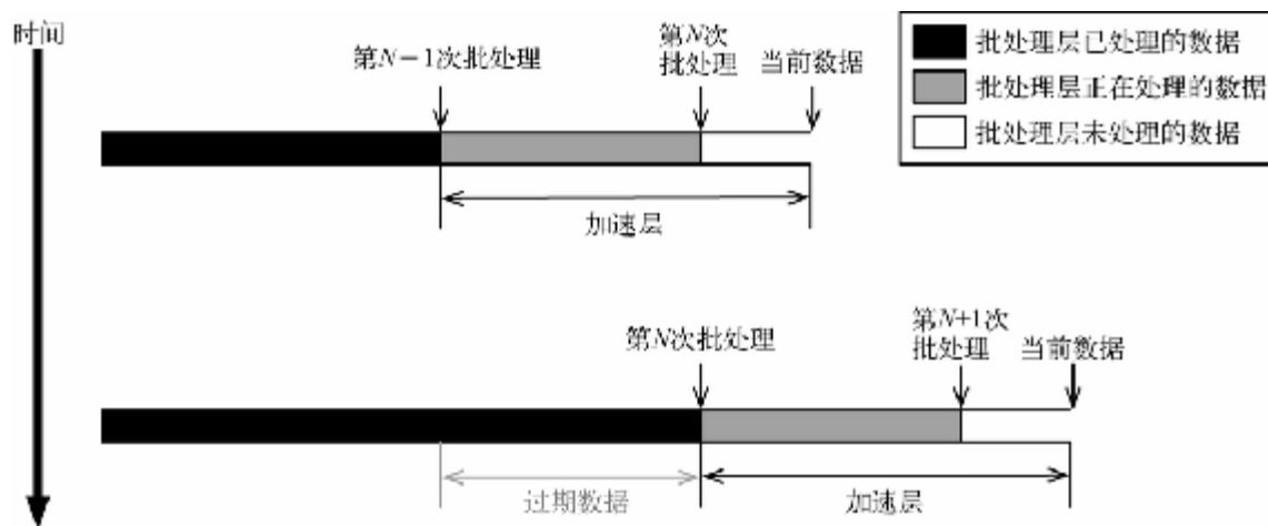
图 8-13 在加速层中让数据过期
