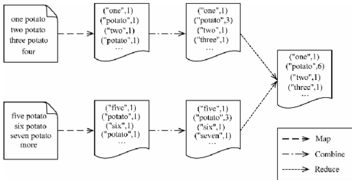
图 8-4 使用combiner
