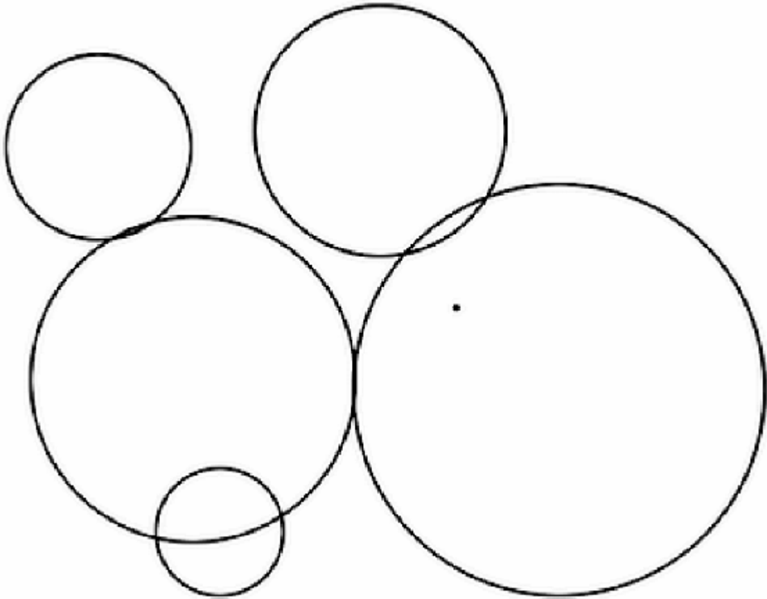
图 6-4 衰减的圆
