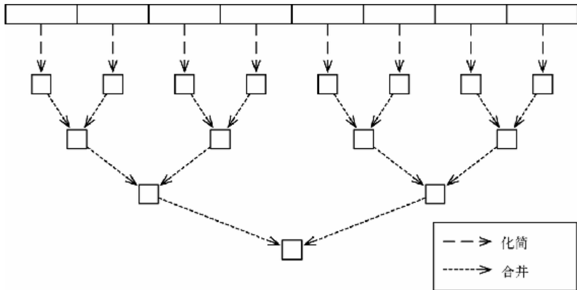
图 3-3 fold 二叉树
