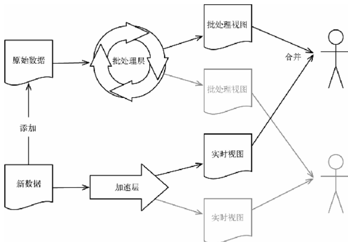
图 8-10 Lambda架构
