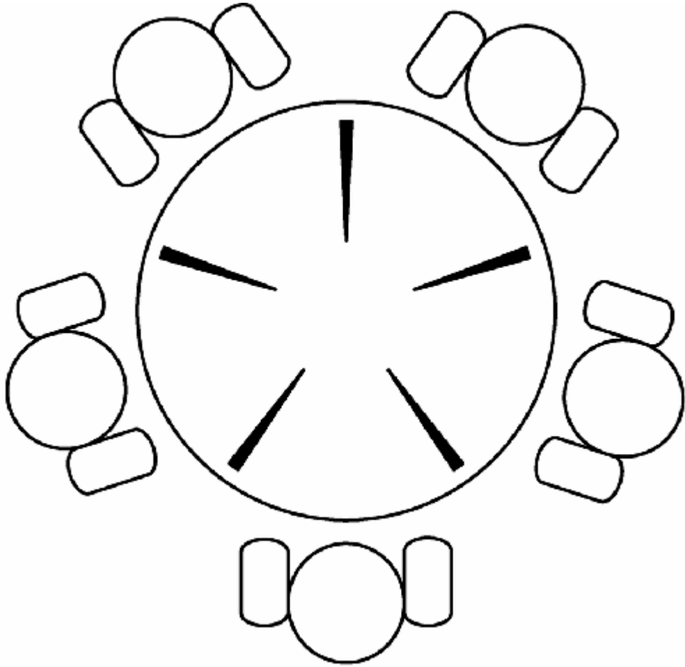
图 2-1 哲学家进餐问题
