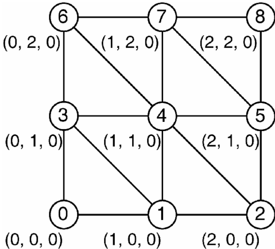
图 7-10 三角形排列成的网格
